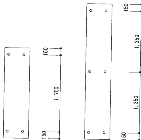
万能板
