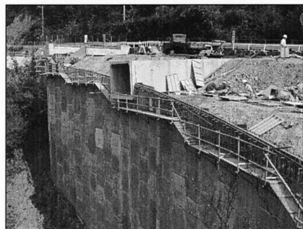
[ テールアルメ・多数アンカー工法 ]
