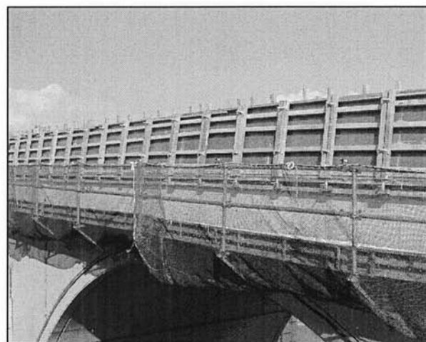
[ テールアルメ・多数アンカー工法 ]
