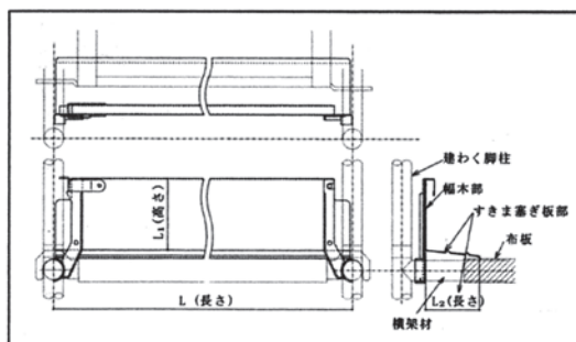
寸法図 建枠横架材取付型
