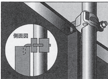
⑤ 最上段はクランプのフックを下向きに 取付ける。
